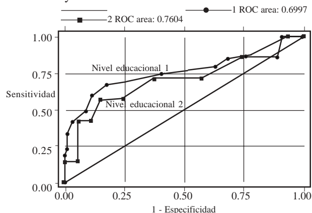
Figura 1. CURVA ROC
